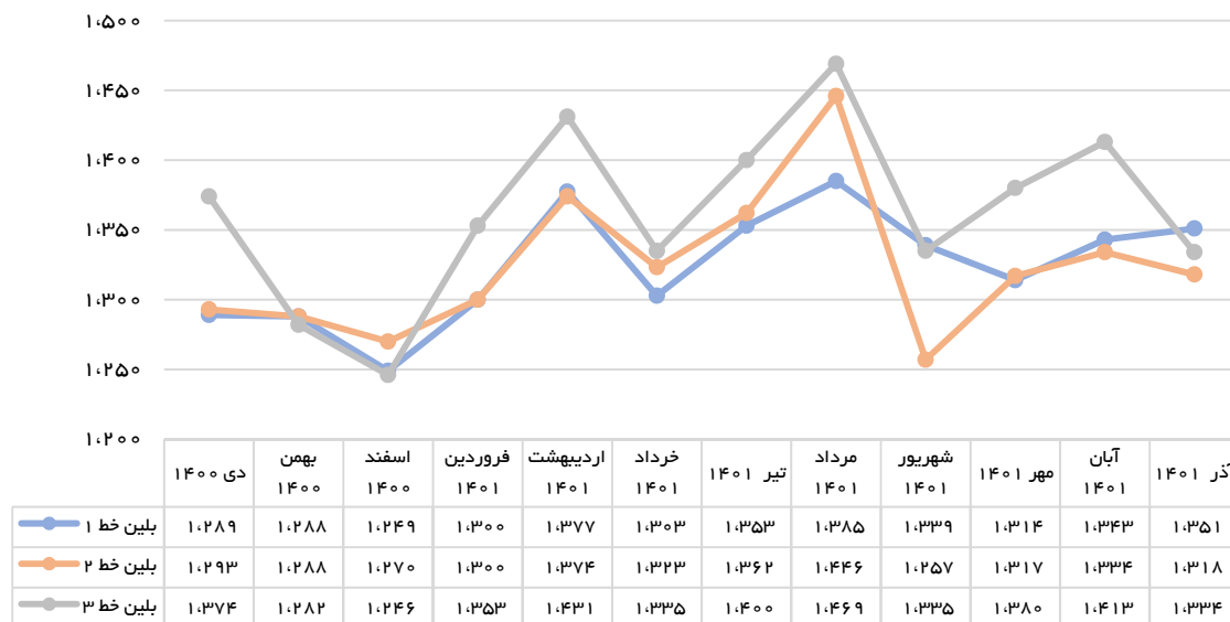
میانگین بلین کنسانتره تولیدی خطوط ۱، ۲ و ۳ طی سال مالی ۱۴۰۱-۱۴۰۰
