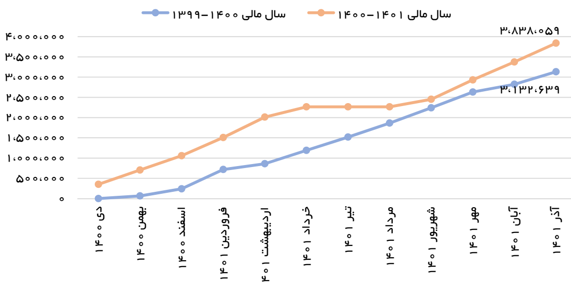
نمودار تجمعی باردهی به کارخانه گندله سازی طی سال های مالی ۱۳۹۹-۱۴۰۰ و ۱۴۰۰-۱۴۰۱
