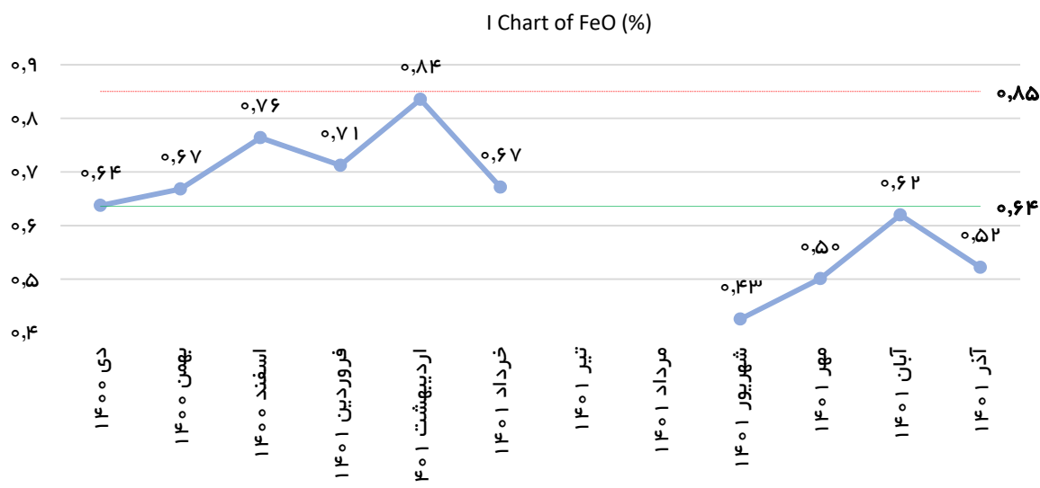
بررسی FeO گندله تولیدی به صورت ماهانه در سال مالی ۱۴۰۰-۱۴۰۱
