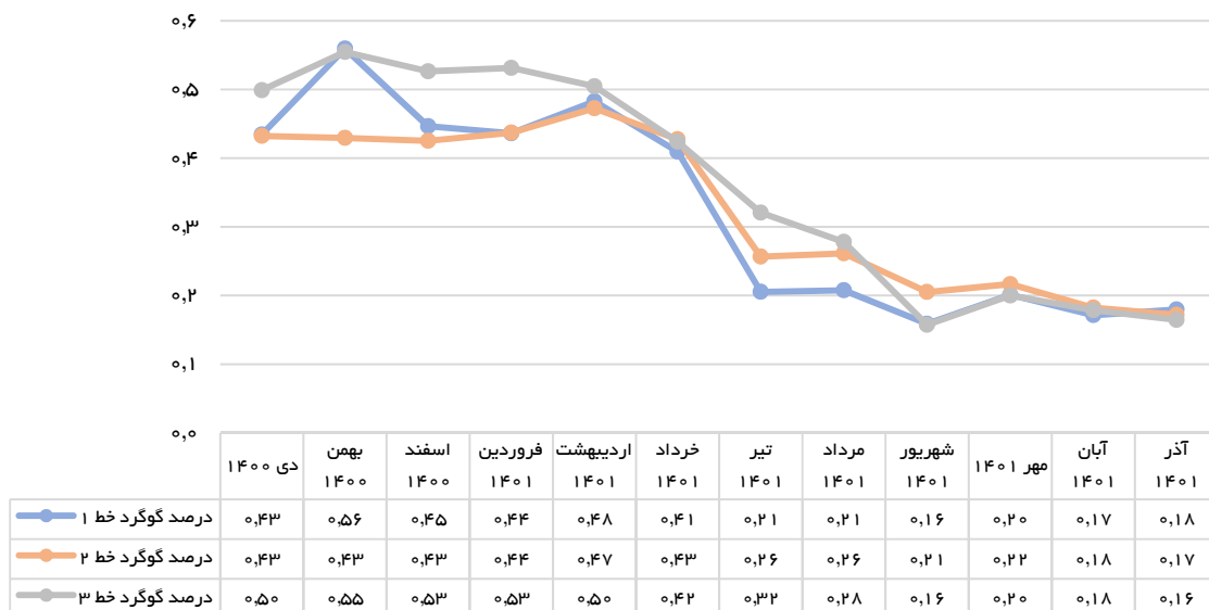
میانگین درصد گوگرد کنسانتره تولیدی خطوط ۱، ۲ و ۳ طی سال مالی ۱۴۰۱-۱۴۰۰
