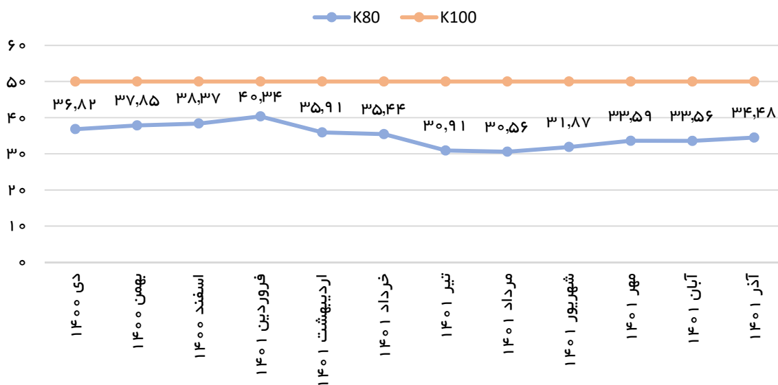
میانگین K80 و K100 سنگ آهن خردایش شده در سال مالی ۱۴۰۱-۱۴۰۰
