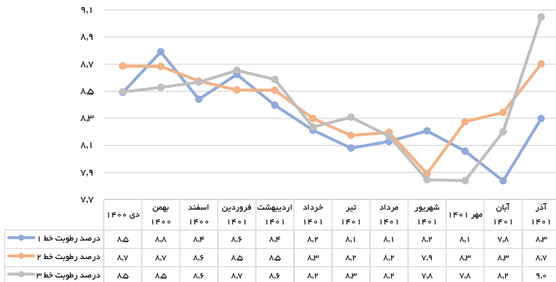
میانگین درصد رطوبت کنسانتره تولیدی خطوط ۱، ۲ و ۳ طی سال مالی ۱۴۰۱-۱۴۰۰
