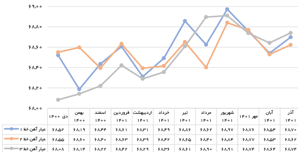
میانگین عیار آهن کنسانتره تولیدی خطوط ۱، ۲ و ۳ طی سال مالی ۱۴۰۱-۱۴۰۰
