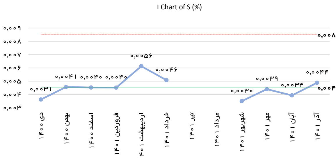
بررسی S گندله تولیدی به صورت ماهانه در سال مالی ۱۴۰۰-۱۴۰۱
